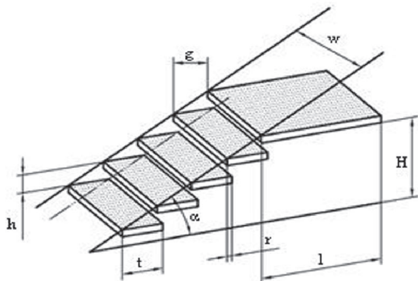
Figura 2: Exemplo de escada sem espelho.
