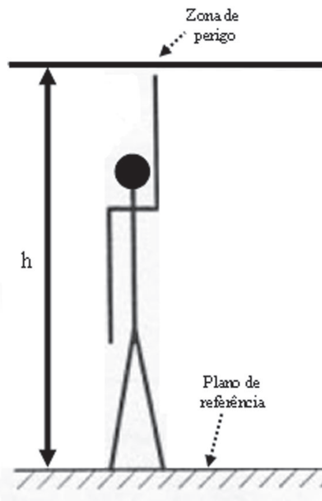
Figura 2 - Alcance das zonas de perigo superiores
